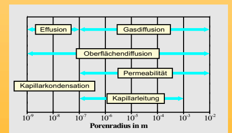
Zusammenhang zwischen verschiedenen Wassertransportmechanismen und den zugehörigen Porenradien [2, 3].
