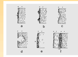
Formen der Salzverwitterung an Wandmalereien (M: Malschicht, P: Putzschicht, S: nadelige Salzkristalle, SK: Salzkruste), nach A. Arnold.
