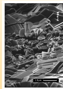
Syngenit-Ausblühungen auf der Oberfläche in Form verschieden geneigter Tafeln.
