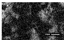
Kalium-Verteilung auf einer mit Syngenit ausgeblühten Modelloberfläche aus Fuji-Hartgips.
