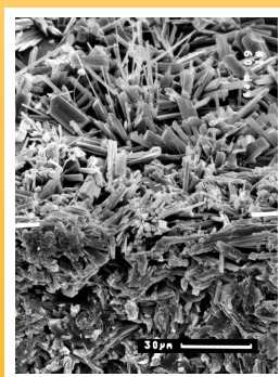
Bruchfläche eines Gipsmodells (Bruchkante markiert). Poren gestatten Lösungstransport. -Ausblühung auf der Oberfläche-
