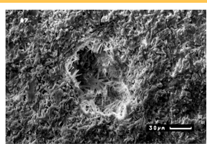
REM-Foto von einer Bruchfläche eines kunststoffvergüteten Gipses. Die Ausblühungen liegen im Inneren einer Blase.
