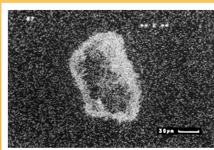
Kalium-Verteilung des Bildausschnitts von links. Die starke Anreicherung des Kaliums in der Blase ist augenfällig.
