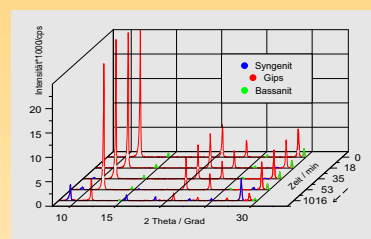
Röntgen-Diffraktogramme einer ausblühenden Gipsoberfläche in zeitlicher Abfolge. Die auftretende Ausblühphase ist Syngenit [ \text{K}_2\text{Ca}(\text{SO}_4)_2 \cdot \text{H}_2\text{O} ].
