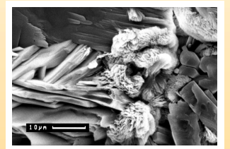
Ein unterschiedlich schneller Transport der Porenlösung ruft verschieden gestaltete Ausblühungen hervor.
