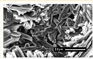
Auf der abgeformten Modelloberfläche (Mitte) zeigt sich vermehrt tafelig ausgebildeter Syngenit (Randbereich).
