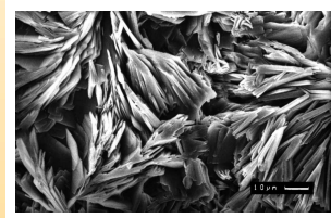
Eine völlig mit Syngenit überzogene Oberfläche. Der Ursprung der Sprossungen deutet auf Porenkanäle hin.
