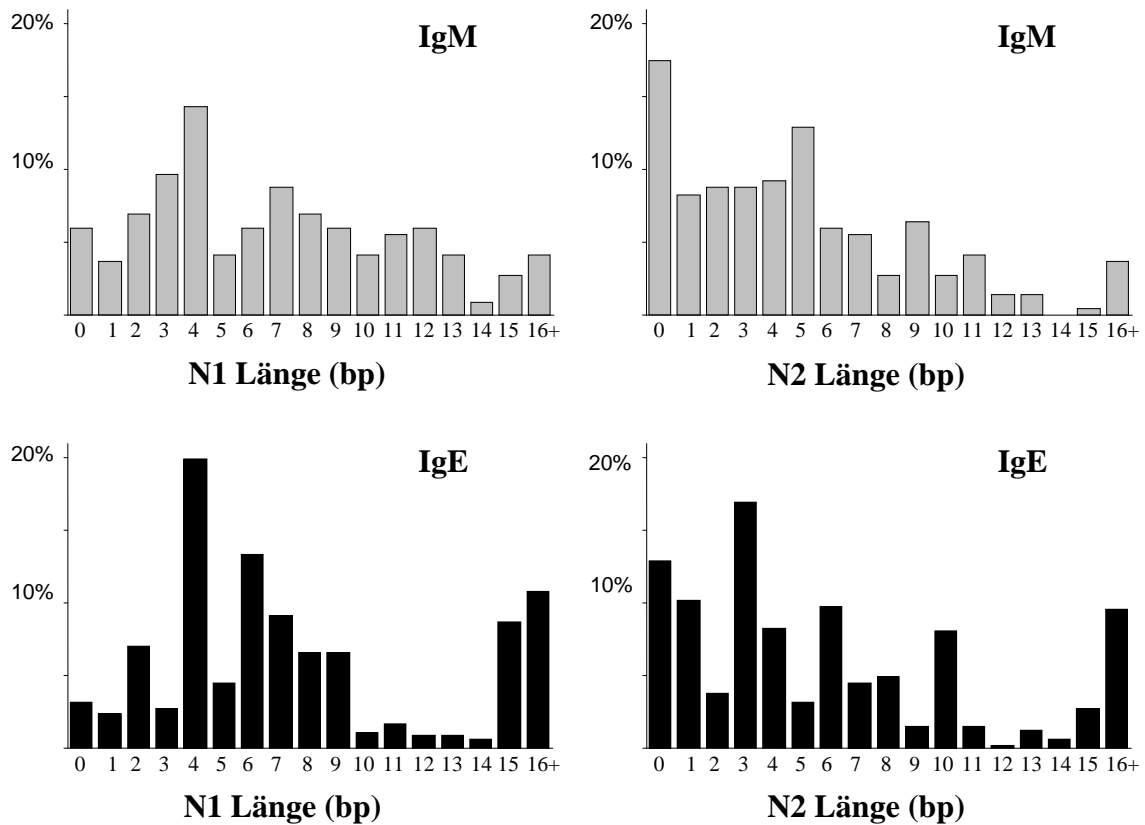
Abbildung 14: Längenverteilung der N-Regionen
