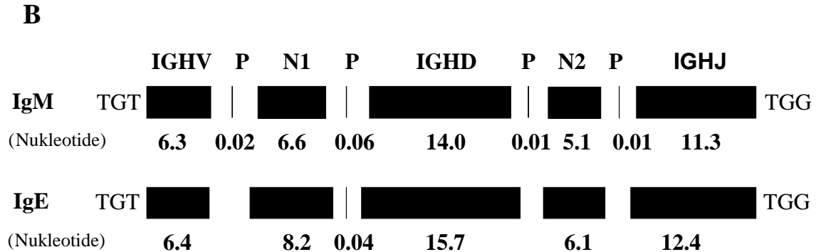
Abbildung 13: Längenverteilung (A) und Zusammensetzung (B) der CDR-H3
