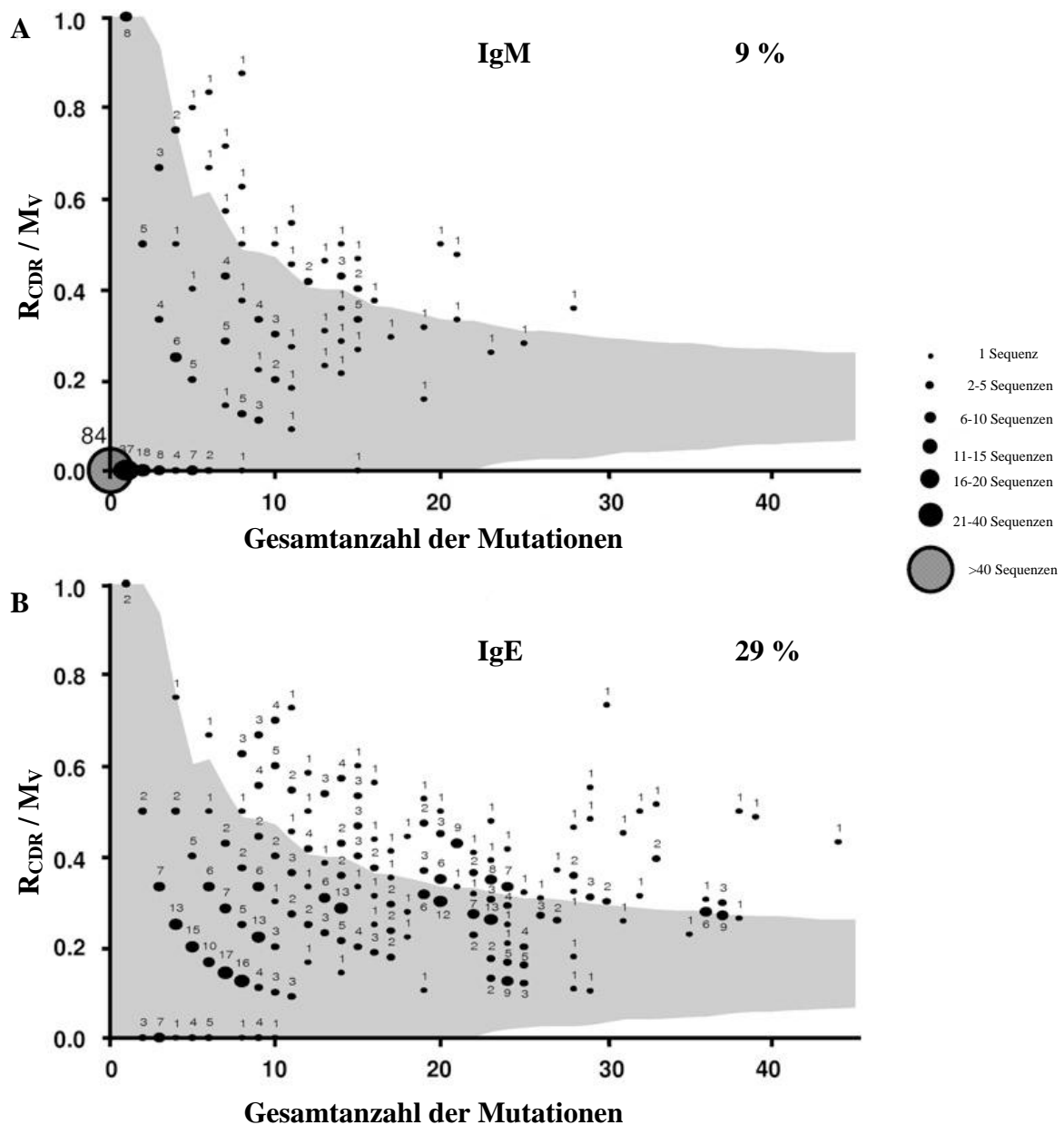
Abbildung 16: Zeichen der Antigenselektion bei IgM- und IgE-Sequenzen
