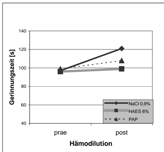
Abb. 3-57 und 3-58 Einfluss der Verdünnung mit NaCl, HAES und PAP auf die Gerinnungszeit bei KC4 (Mittelwerte, n=10 ) und SGC (Mittelwerte, n=15 )
