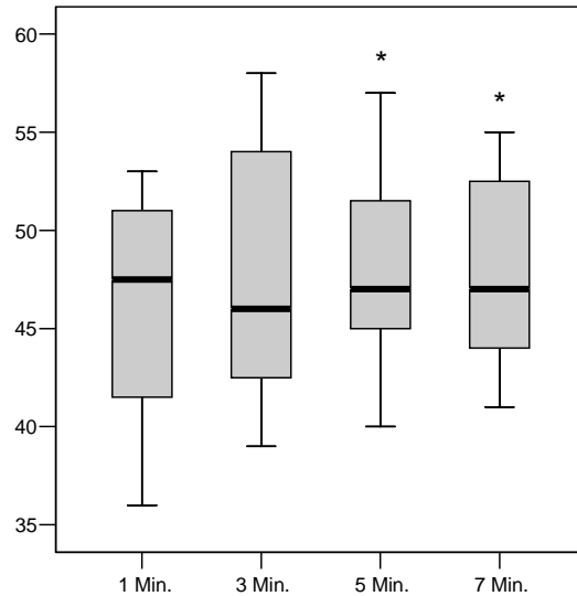
Abb. 3-18 MCF in NATEM mit Citratblut
