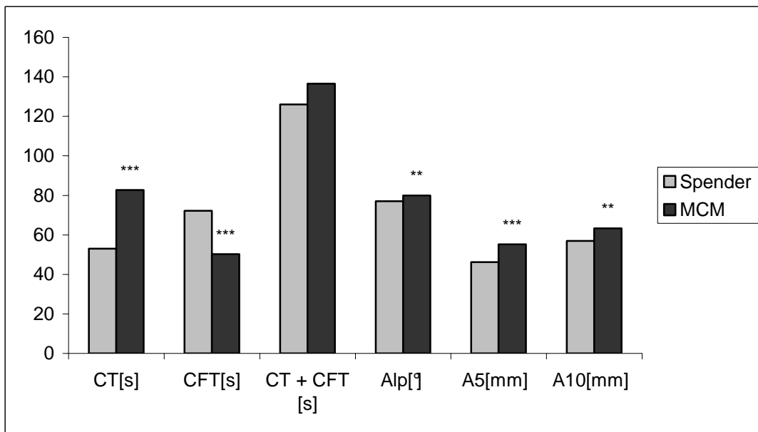
Abb. 3-65 Diaplastin - Medianwerte der Parameter bei Pat. mit Marcumar im Vergleich mit Spendern
