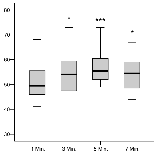
Abb. 3-8 CT in EXTEM mit Citratblut
