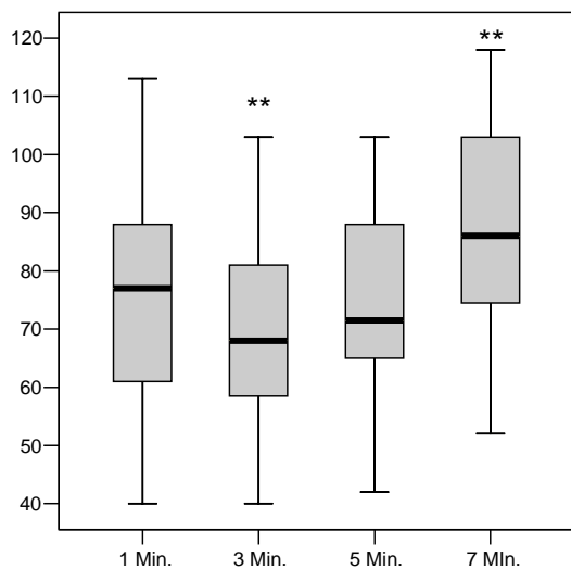
Abb. 3-3 CFT in INTEM mit Nativblut
