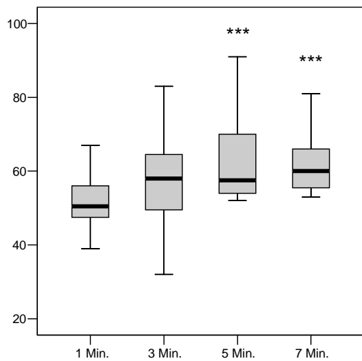
Abb. 3-7 CT in EXTEM mit Nativblut
