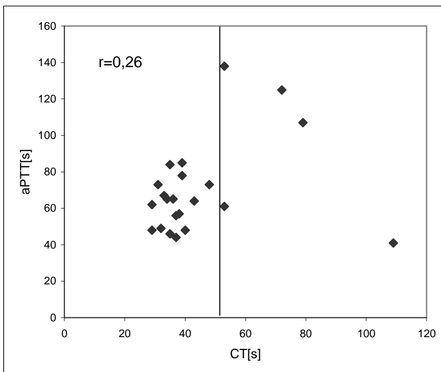
Abb. 3-63 EXTEM - Korrelation zwischen CT und aPTT bei Patienten mit Heparin, n=22
