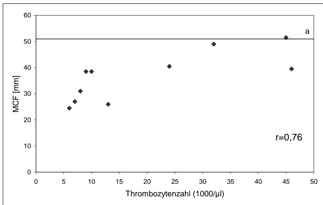
Abb. 3-61 Korrelation zwischen MCF/INTEM und der Thrombozytenzahl (n=10 Patienten)
