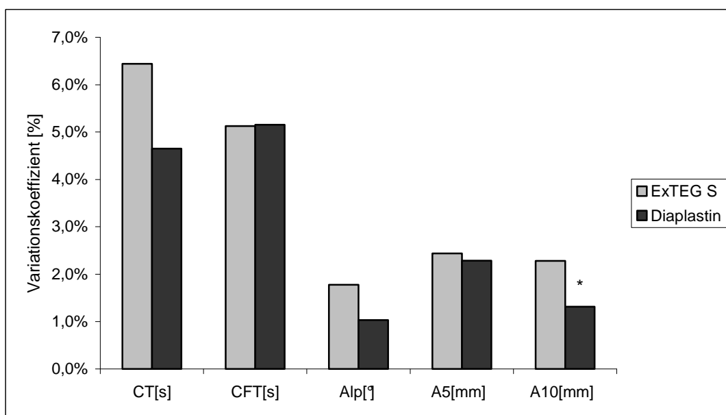
Abb. 3-84 Intensivpatienten, VK der Parameter, ExTEG S vs. Diaplastin, n=22
