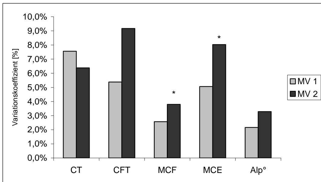
Abb. 3-37 Variationskoeffizienten V_k in EXTEM bei unterschiedlichen Pipettierverfahren (Mischverfahren)
