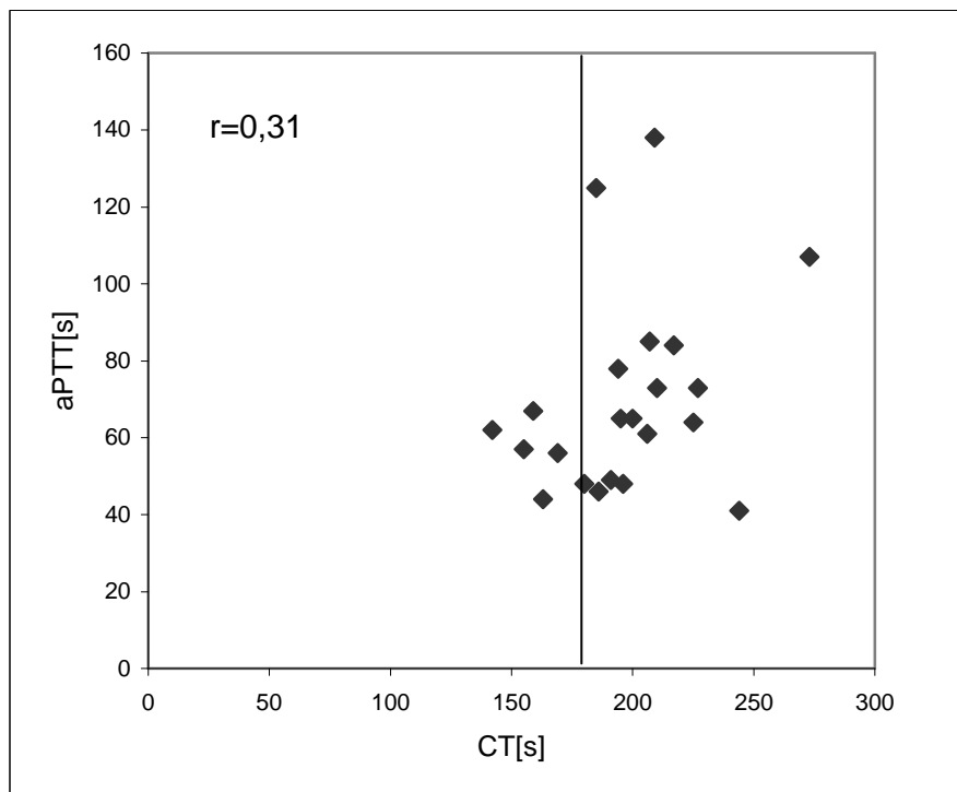
Abb. 3-62 INTEM - Korrelation zwischen CT und aPTT bei Patienten mit Heparin, n=22
