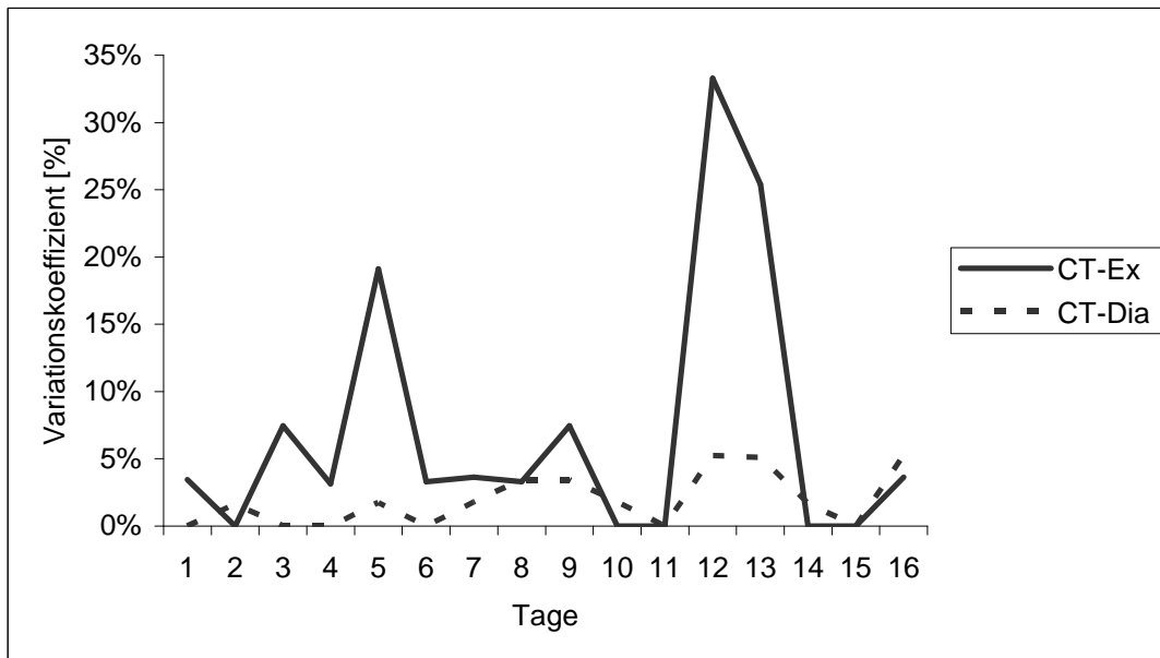
Abb. 3-43 Variationskoeffizienten V_k für die CT von Doppelbestimmungen mit ROTROL bei Verwendung von EXTEG S und Diaplastin als Aktivatorreagenzien über 16 Tage
