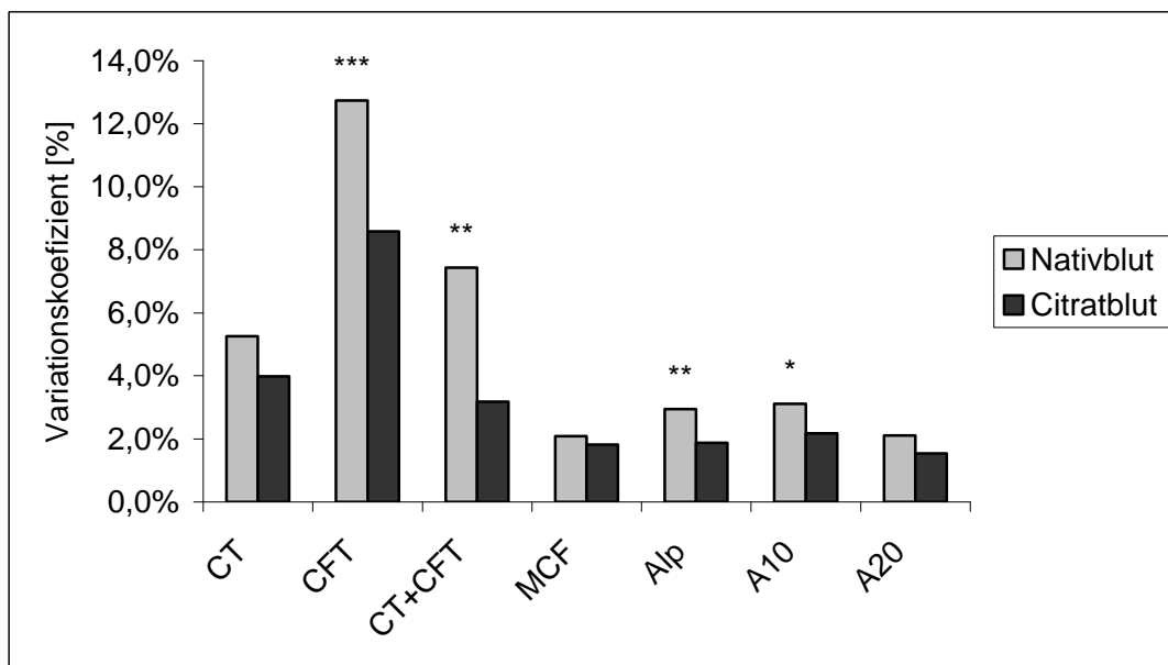
Abb. 3-30 Nativblut vs. Citratblut, Medianwerte der V k bei INTEM, Spender, n=20
