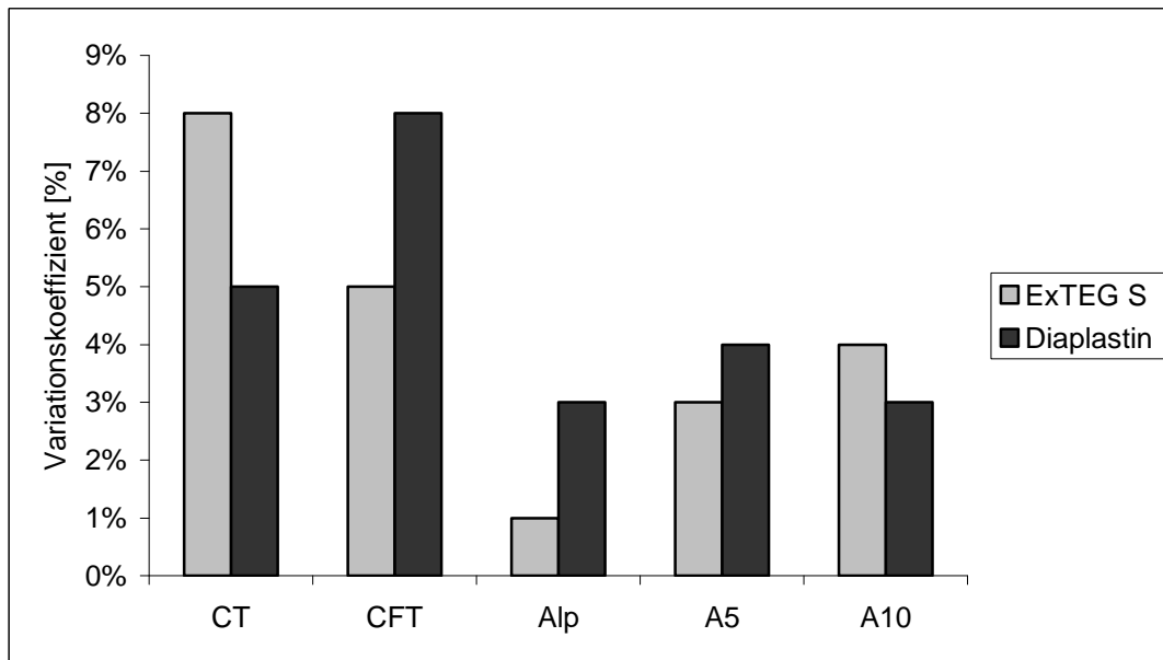
Abb. 3-69 Variationskoeffizienten für Doppelbestimmungen von EXTEM mit zwei verschiedenen Aktivatorreagenzien bei Patienten (n=8) mit erhöhten Leberwerten
