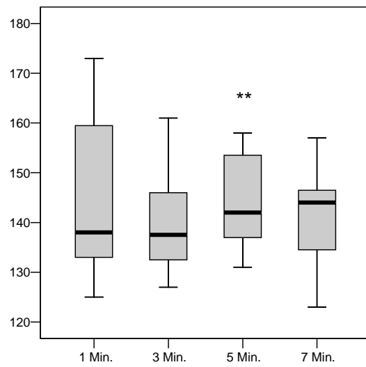
Abb. 3-2 CT in INTEM mit Citratblut
