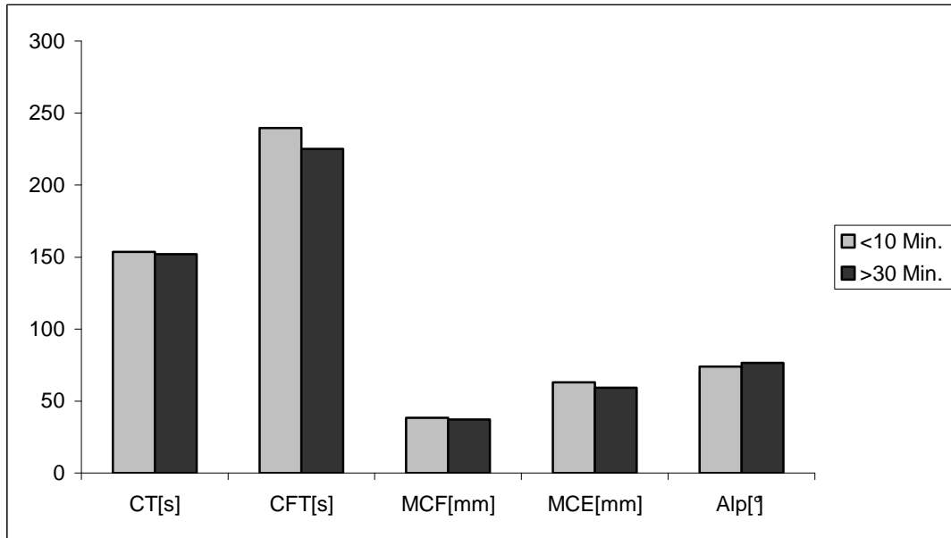
Abb. 3-23 INTEM Parameter bei Untersuchung von Citratblut 10 und 30 Min. nach Blutentnahme, (Medianwerte, Patienten mit Thrombozytopenie, n=10)
