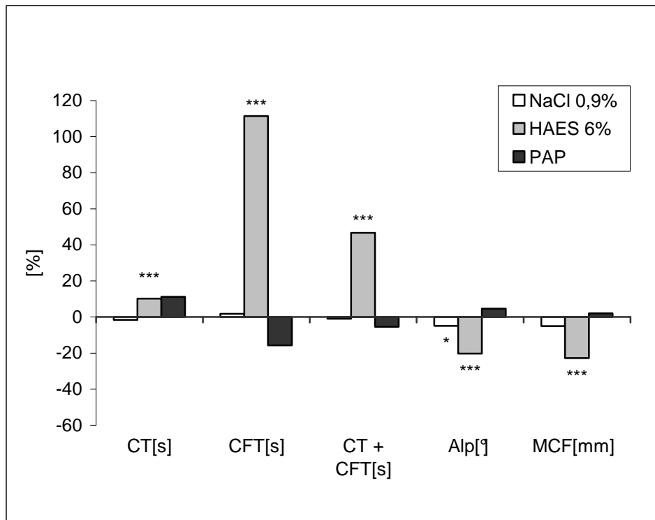
Abb. 3-61 Mittlere Veränderungen [%] der INTEM-Parameter bei Hämodilution mit NaCl, HÄS und PAP von 10 Messreihen
