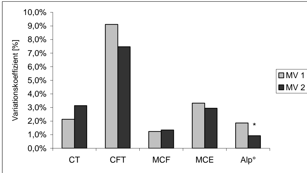
Abb. 3-36 Variationskoeffizienten V_k in INTEM bei unterschiedlichen Pipettierverfahren (Mischverfahren, MV)
