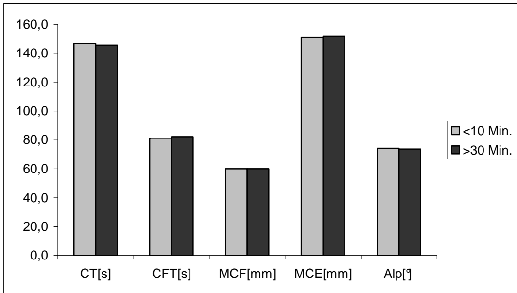
Abb. 3-19 INTEM Parameter bei Untersuchung von Citratblut 10 und 30 Min. nach Blutentnahme, (Medianwerte, Spender, n=10)
