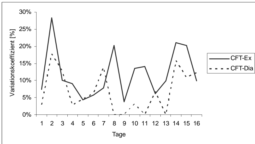
Abb. 3-44 Variationskoeffizienten V_k für die CFT von Doppelbestimmungen mit ROTROL bei Verwendung von EXTEG S und Diaplastin als Aktivatorreagenzien über 16 Tage
