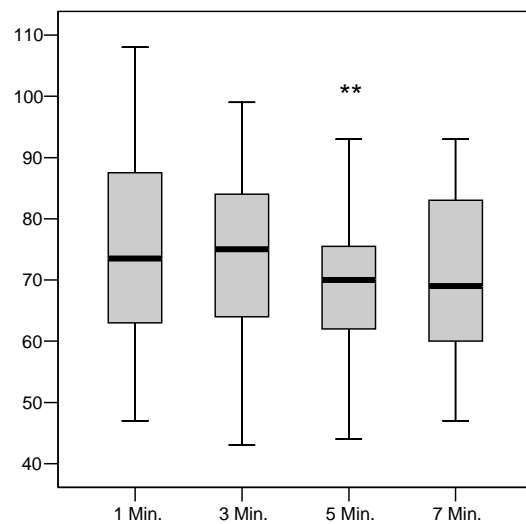
Abb. 3-4 CFT in INTEM mit Citratblut
