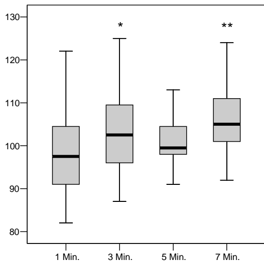
Abb. 3-1 CT in INTEM mit Nativblut
