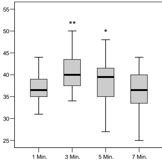
Abb. 3-17 MCF in NATEM mit Nativblut
