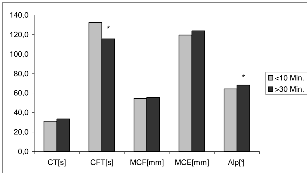
Abb. 3-20 EXTEM Parameter bei Untersuchung von Citratblut 10 und 30 Min. nach Blutentnahme, (Medianwerte, Spender, n=10)
