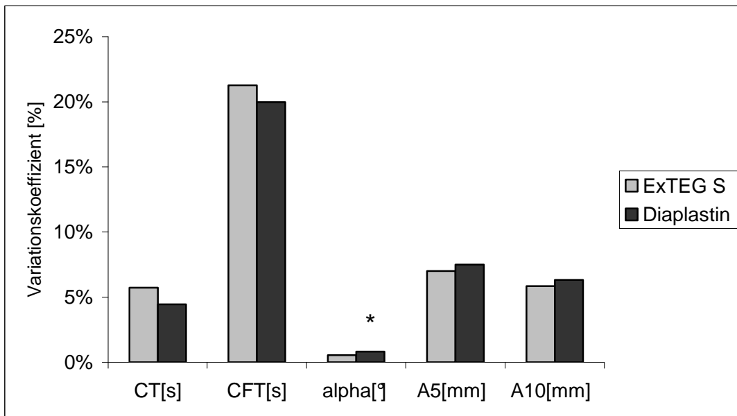
Abb. 3-40 Variationskoeffizienten ( V_k ) der Messergebnisse mit ROTROL bei 10 auf einander folgenden Messungen (Mittelwerte) unter Verwendung von ExTEG S und Diaplastin als Aktivatorreagenzien
