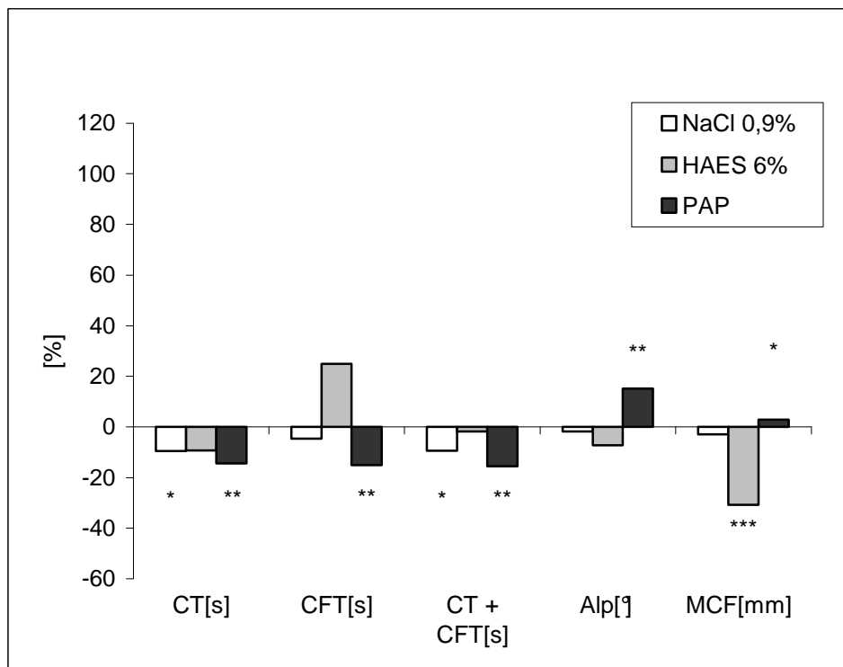
Abb. 3-60 Mittelwerte der Differenzen, vor und nach Hämodilution, aus Messreihe 1-10 in %, NATEM
