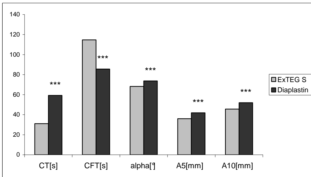
Abb. 3-41 Vergleich der Messergebnisse mit Spenderblut bei 10 aufeinander folgenden Messungen (Mittelwerte) unter Verwendung von ExTEG S und Diaplastin als
