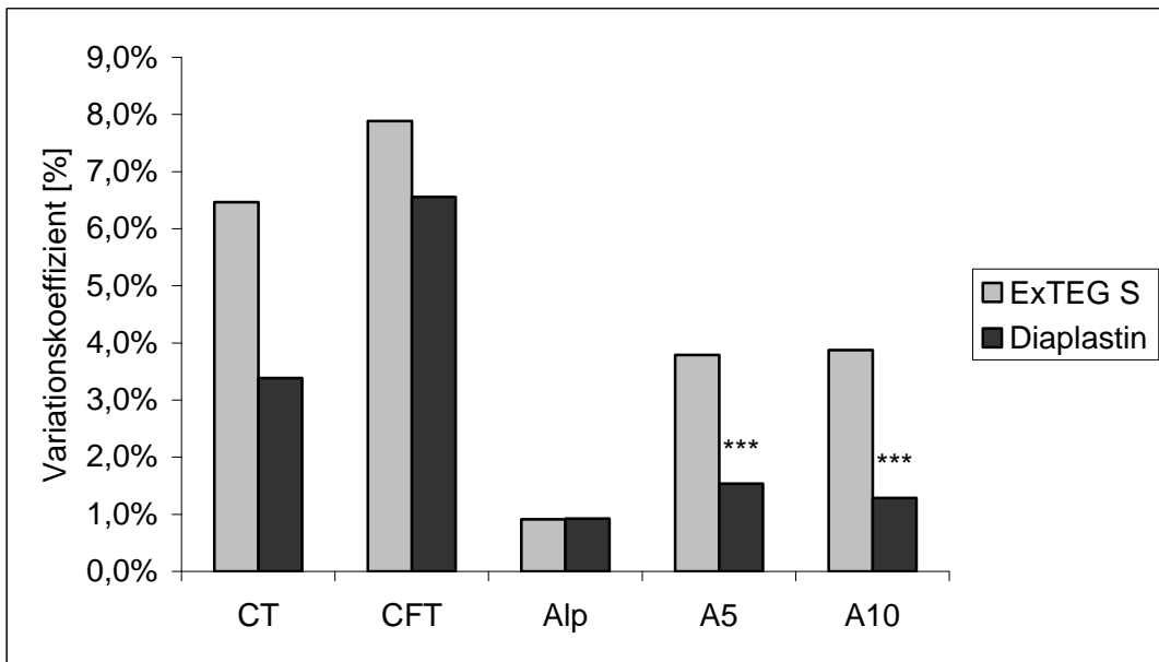
Abb. 3-66 Orale Antikoagulation, VK der Parameter, ExTEG S vs. Diaplastin, n=38
