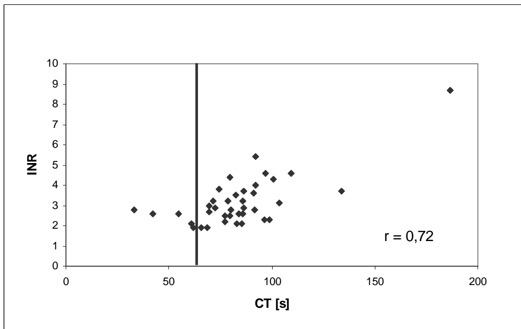
Abb. 3-68 Korrelation von EXTEM-CT bei Verwendung von Diaplastin mit der INR bei Patienten unter Marcumar (n=38)
