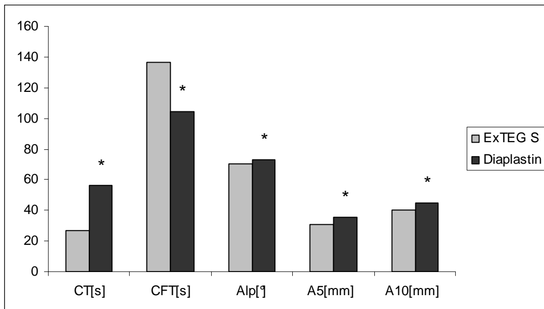
Abb.3-68 EXTEM-Ergebnisse (Mediane) mit zwei verschiedenen Aktivatorreagenzien bei Pat. mit erhöhten Leberwerten (n = 8)
