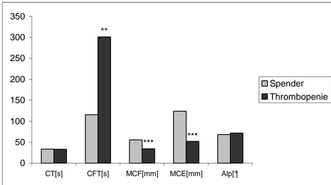
Abb. 3-67 EXTEM Parameter bei Proben von Patienten mit Thrombozytopenie im Vergleich zu solchen von gesunden Blutspendern (n=10)
