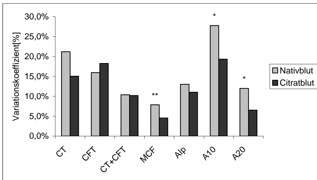
Abb. 3-32 Nativblut vs. Citratblut, Medianwerte der V_k bei NATEM, Spender, n=20
