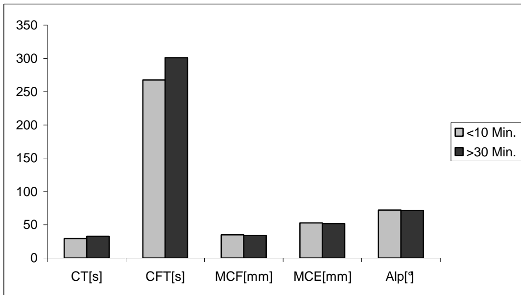
Abb. 3-24 EXTEM Parameter bei Untersuchung von Citratblut 10 und 30 Min. nach Blutentnahme, (Medianwerte, Patienten mit Thrombozytopenie, n=10)
