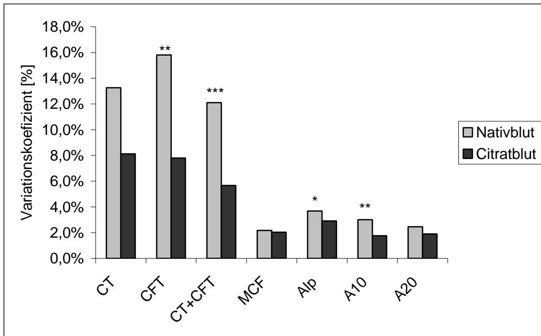
Abb. 3-31 Nativblut vs. Citratblut, Medianwerte der V_k bei EXTEM, Spender, n=20
