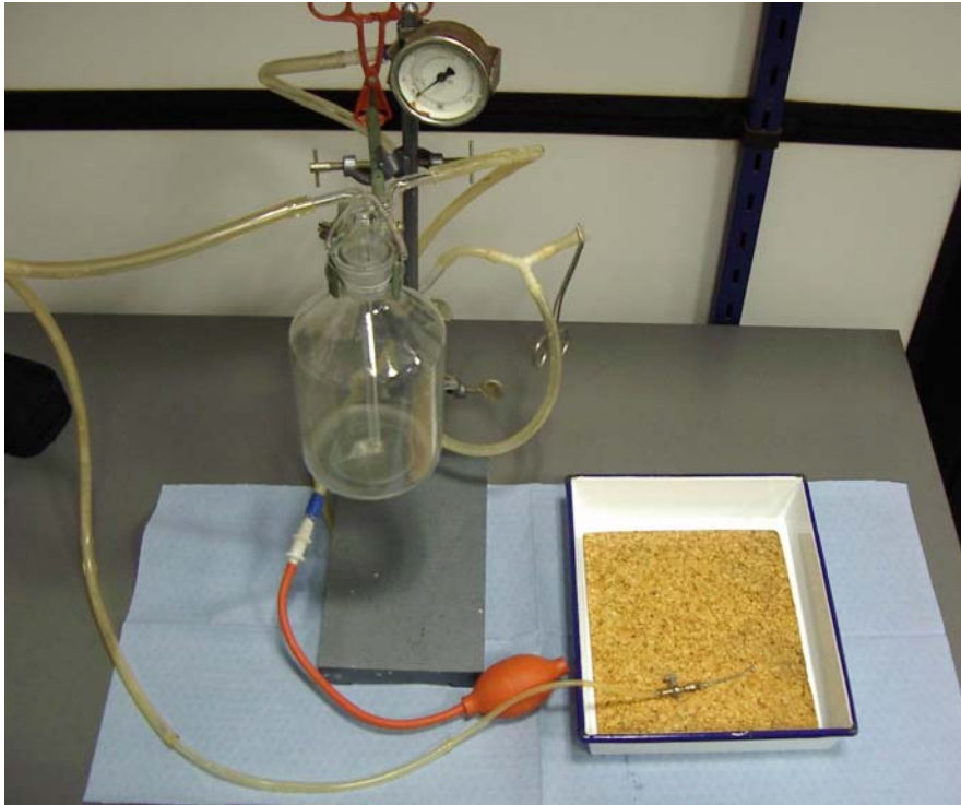
Abbildung 4: Perfusionssystem zur intravitalem Perfusion
